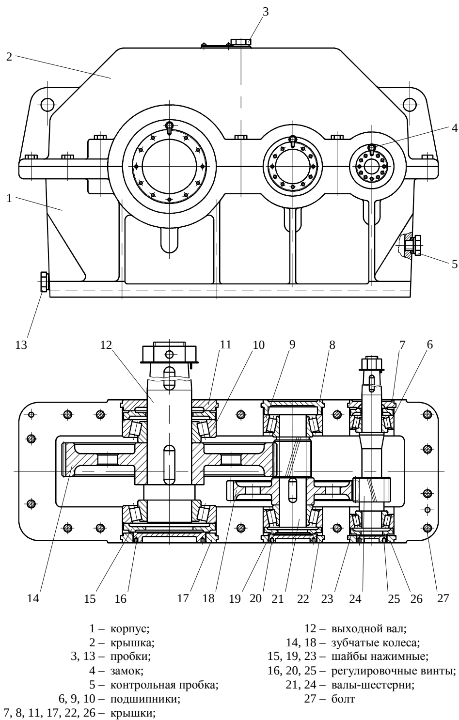
Рисунок 3.12 – Редуктор
