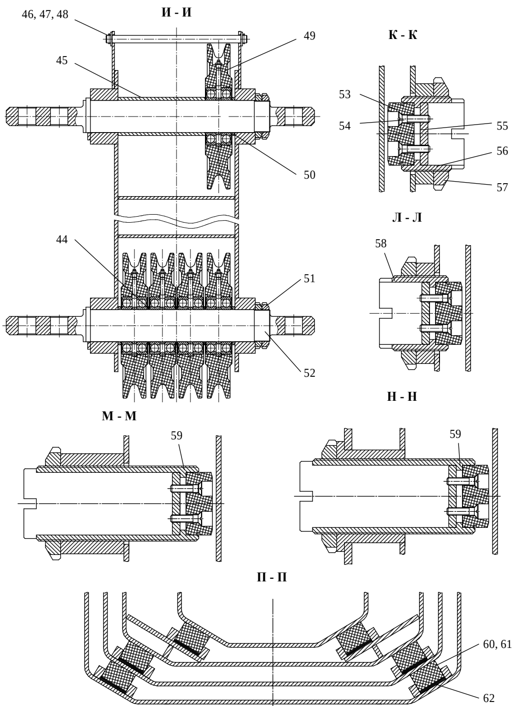
Рисунок 3.17.4 - Стрела телескопическая
