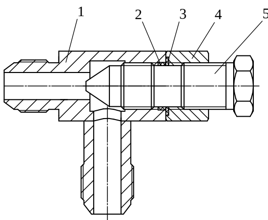
Дроссель ДР6
