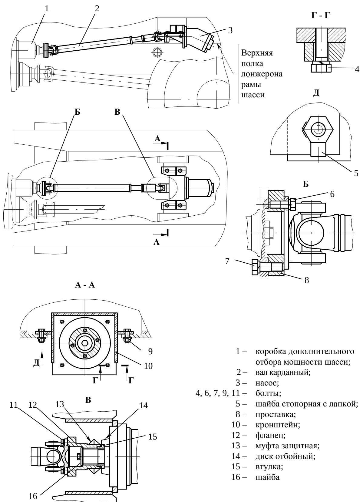
Рисунок 2.6 – Привод насоса
