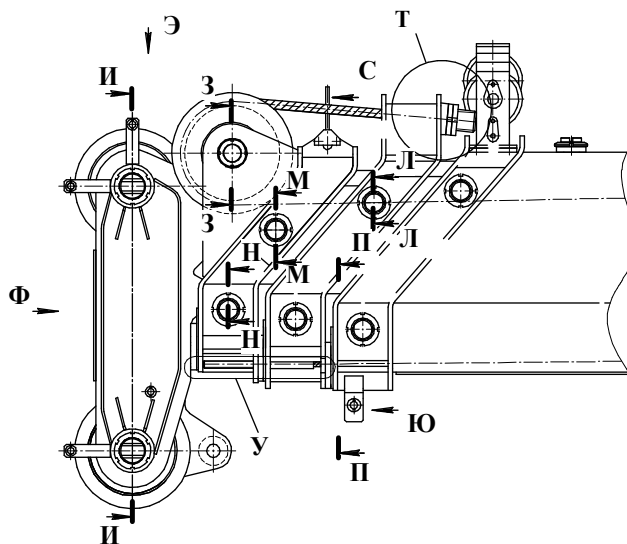
Рисунок 3.17.2 - Стрела телескопическая
