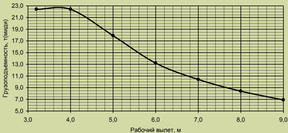
Грузовая характеристика. Лст=9,9-11,0м. \kappa=10 противовес G=1,7 т.
