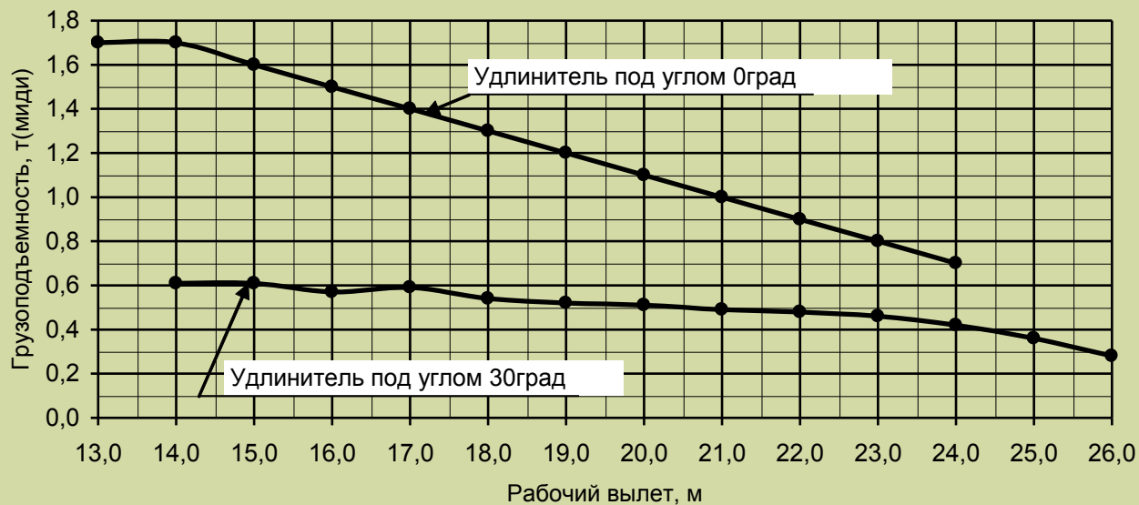
Грузовая характеристика. Лст=30,7м. κ=1. Установлен удлинитель. Противовес G=1,7 т.
