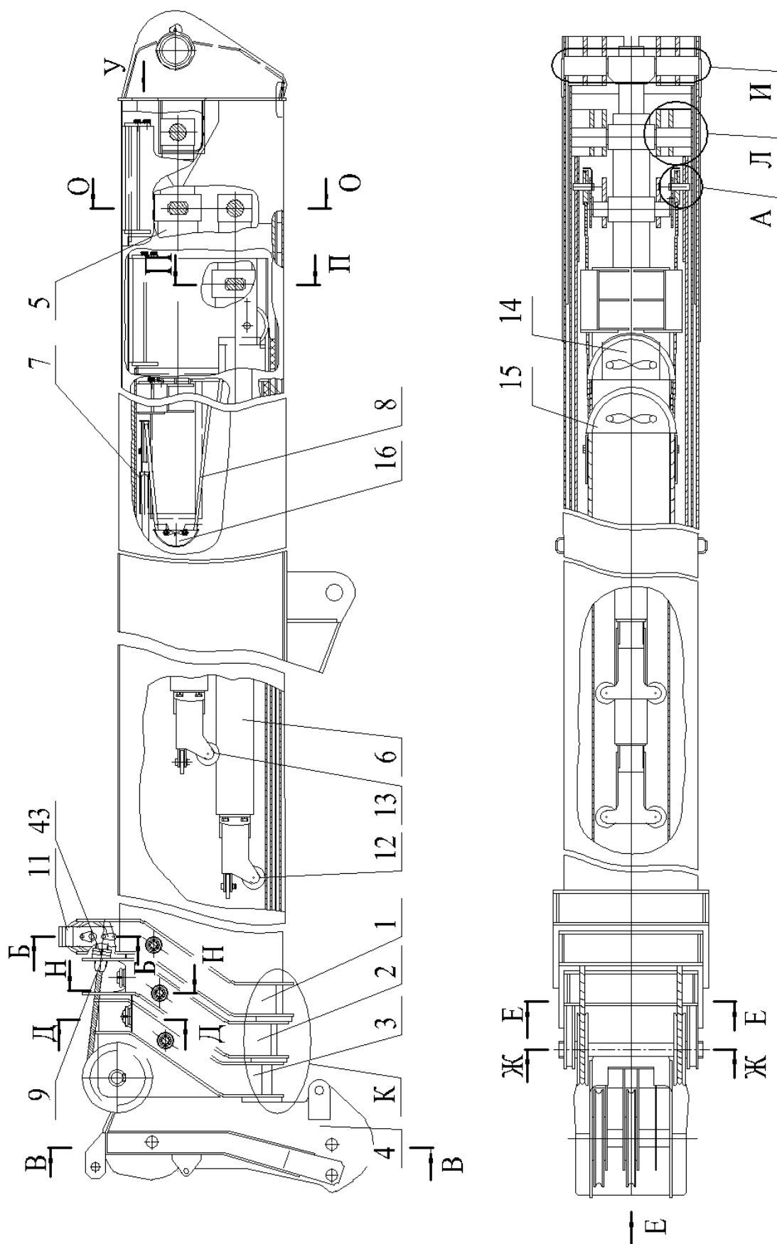
Рисунок 19 Стрела телескопическая
