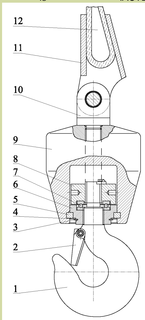
1 – крюк; 2 – защелка; 3 – кольцо; 4 – шайба; 5 – сухарь; 6 – опора; 7 – подшипник; 8 – гайка; 9 – груз; 10 – тяга; 11 – втулка клиновья; 12 - клин
