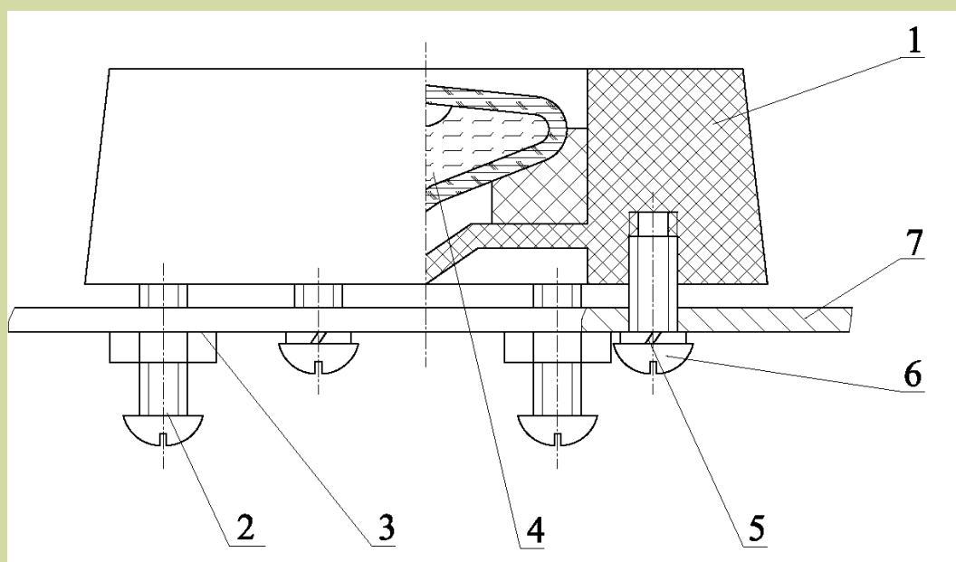
1 – корпус; 2,6 – винты; 3 – гайка; 4 – ампула АНК60-44 ГОСТ 2386-73; 5 – шайба пружинная; 7 - кронштейн
