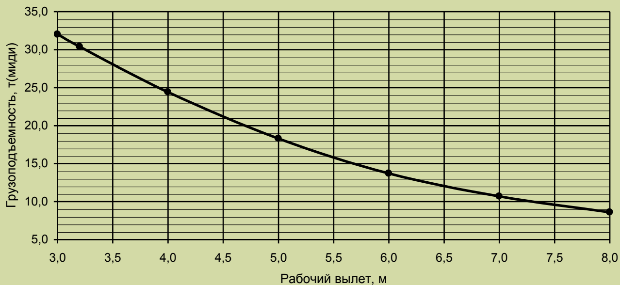
Грузовая характеристика. Лст=9,9м. \kappa=12 , противовес G=1,7 т.
