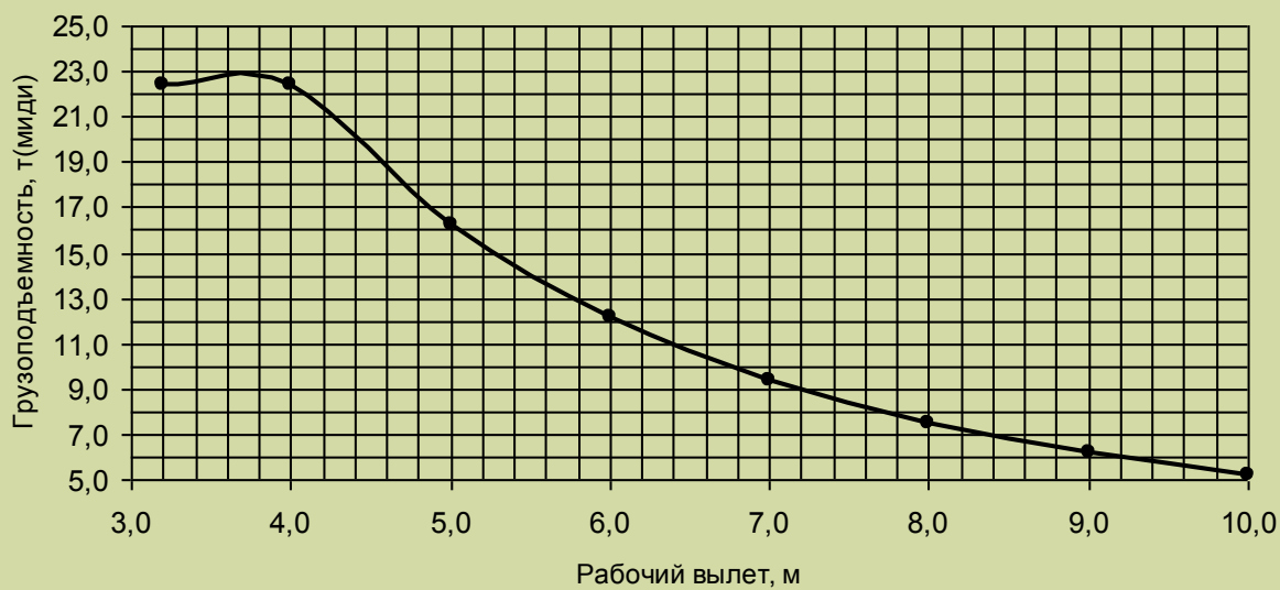
Грузовая характеристика. Лст=11,0-12,0м. \kappa=10 противовес G=1,7 т.
