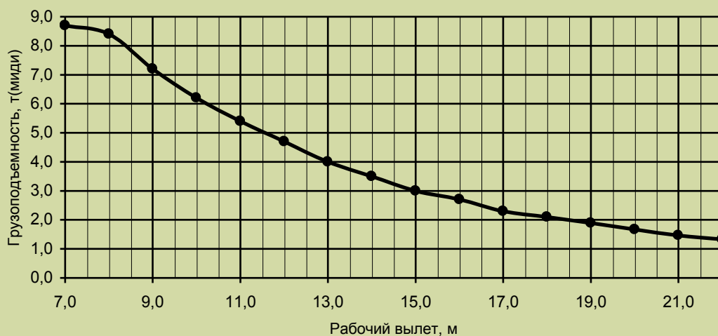
Грузовая характеристика. Лст=22,0-24,0м. \kappa=4 , противовес G=4,2 т.
