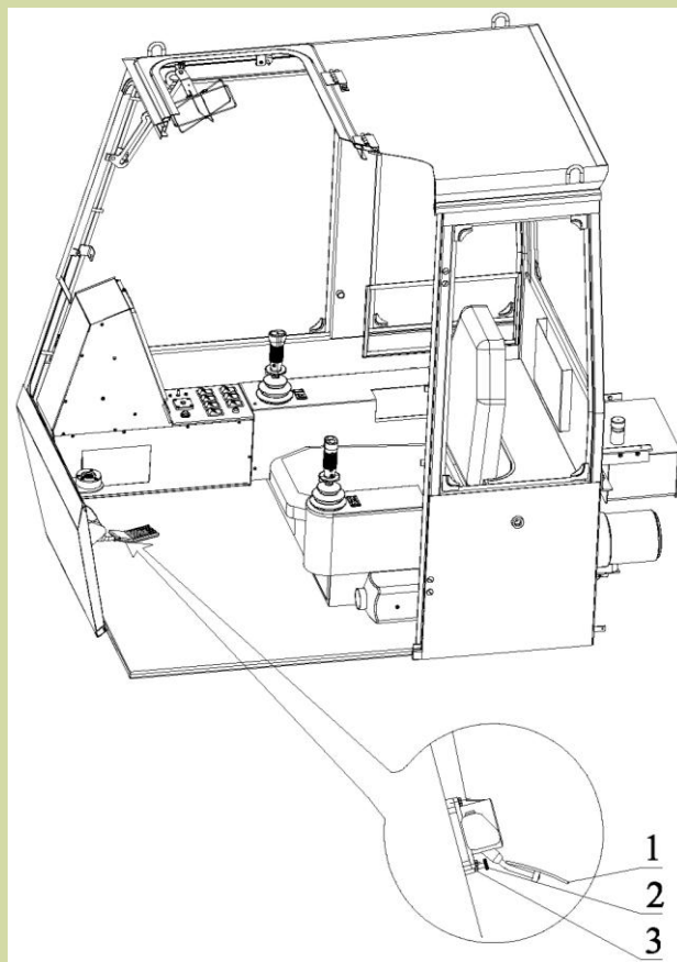
1- педаль управления топливоподачей; 2- винт; 3- контргайка.
