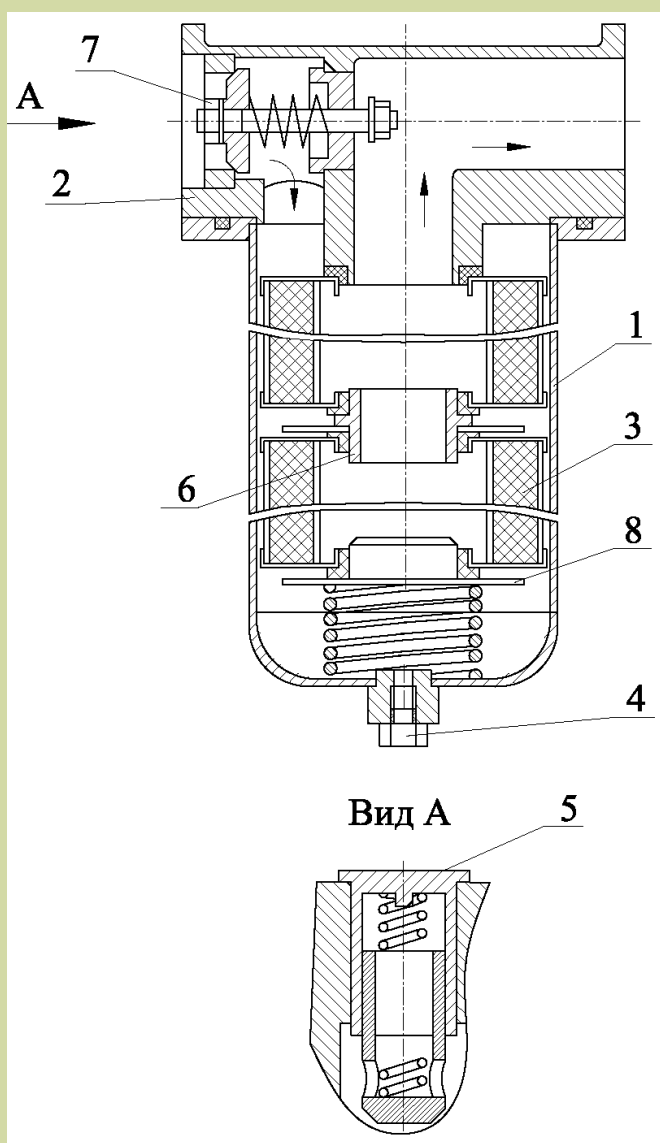
1 - корпус; 2- крышка; 3- фильтроэлемент; 4- пробка; 5- предохранительный клапан; 6- шайба промежуточная; 7- запорное устройство; 8- поддон
