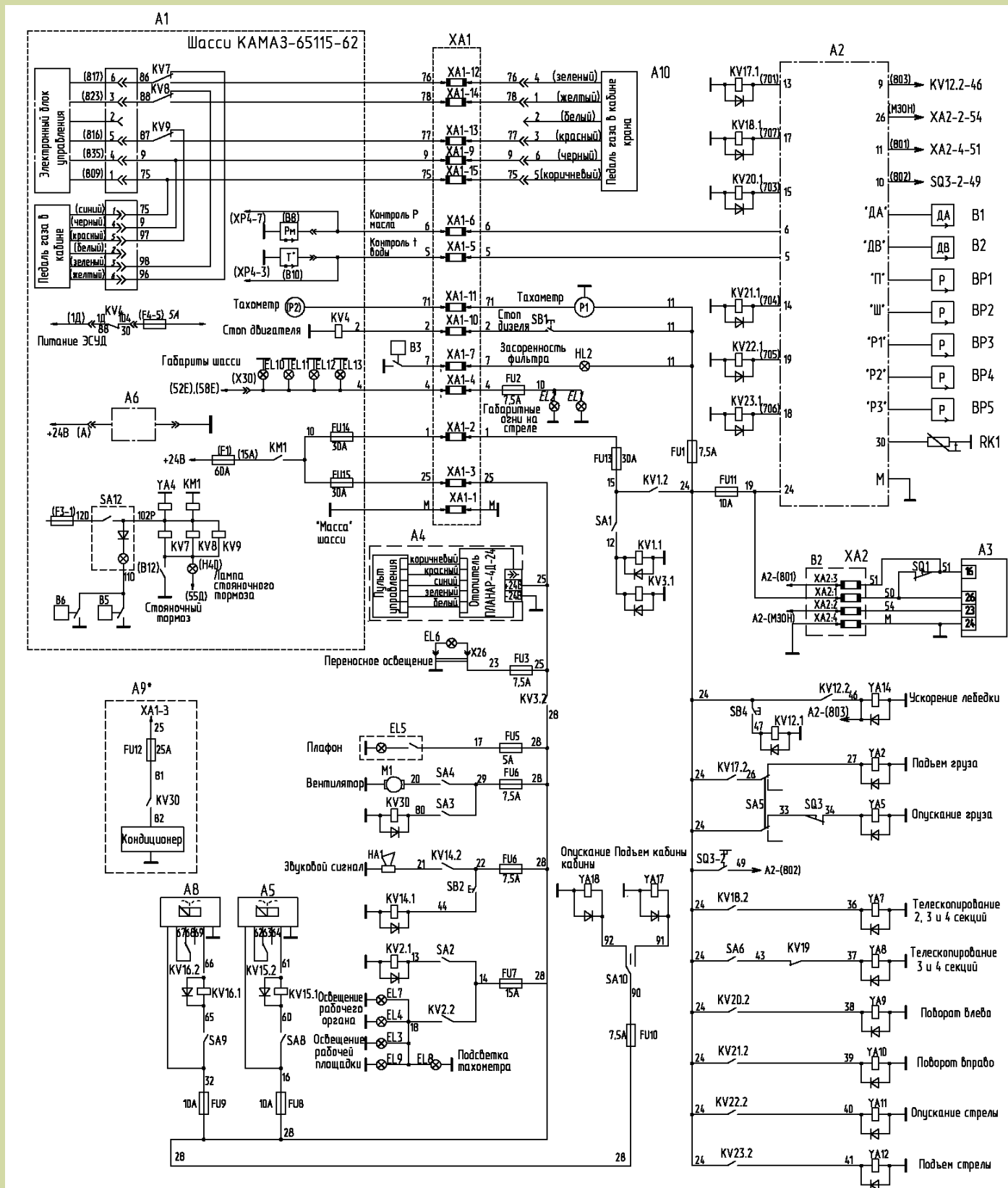
Рисунок 27 Схема электрическая принципиальная (шасси KAMA3-65115-62)
