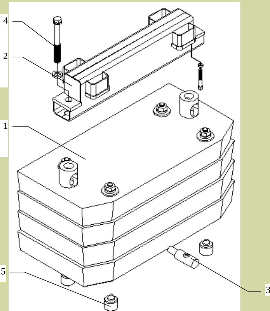
1 – противовес; 2 – балка; 3 – палец; 4 – болт; 5 – установочный выступ
