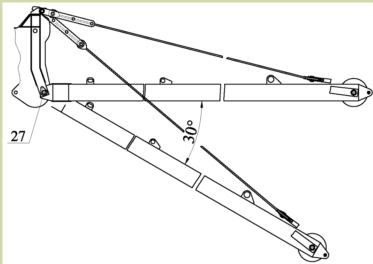
27- палец
