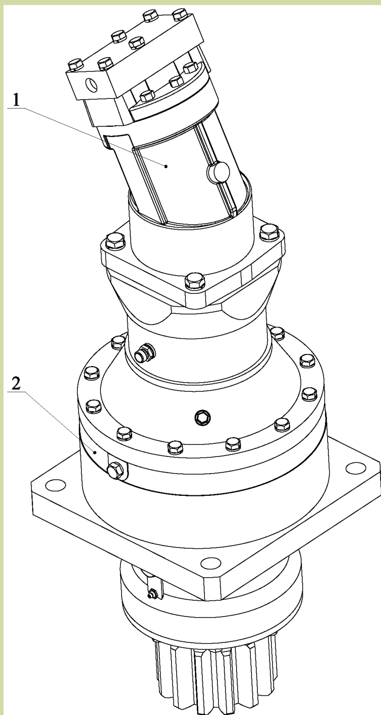
Рисунок 16 Механизм поворота
