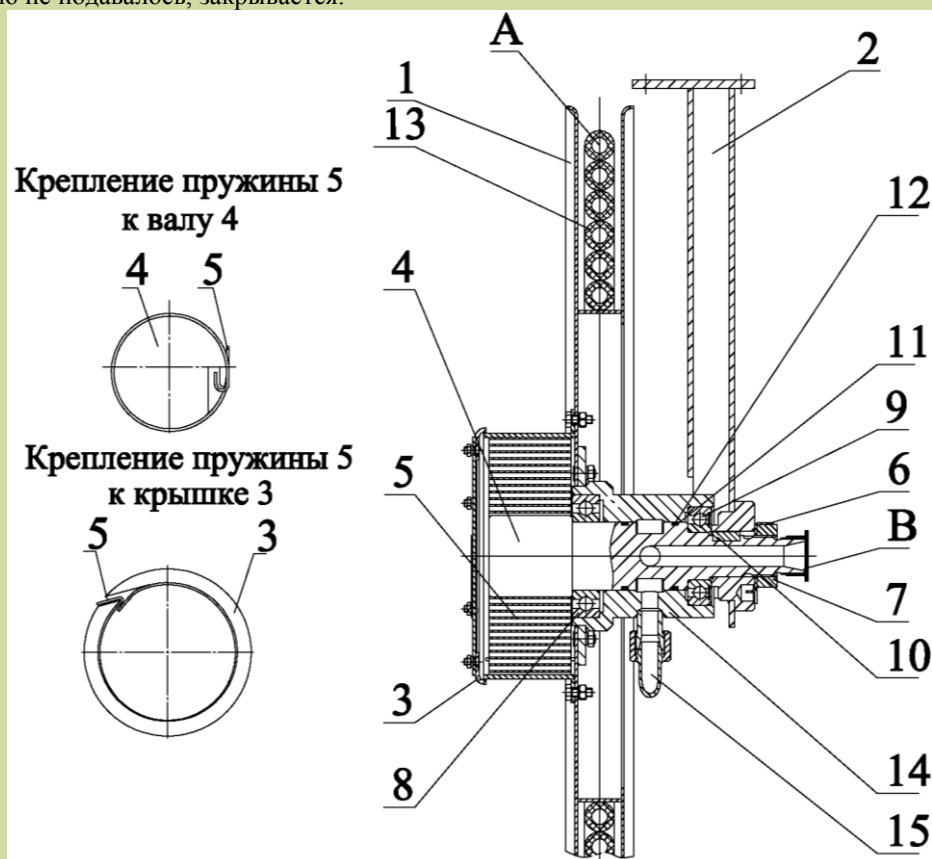
1- барабан; 2- кронштейн; 3- крышка; 4- вал; 5- пружина; 6- шайба стопорная; 7- гайка; 8,9- подшипник; 10- шпонка; 11- кольцо защитное; 12- кольцо; 13- РВД; 14- ступица барабана; 15- трубка. А- к гидроцилиндру; В- к гидрораспределителю
