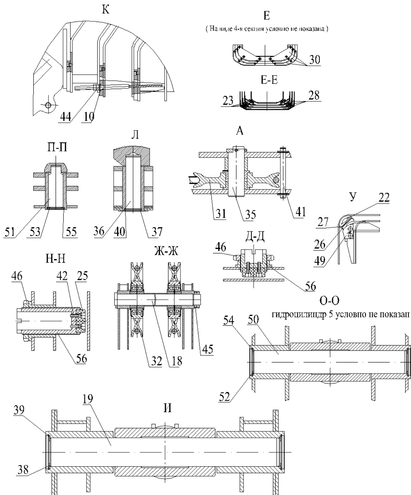
Рисунок 19.1 Стрела телескопическая
