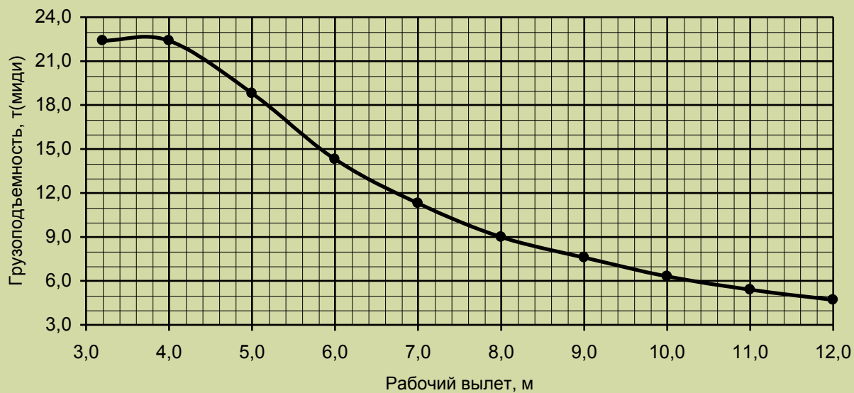
Грузовая характеристика. Лст=12,0-14,0м. \kappa=10 , противовес G=4,2 т.
