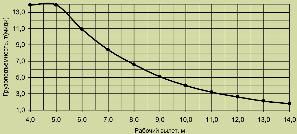
Грузовая характеристика. Лст=16,7-18,0м. \kappa=4 , противовес G=1,7 т.
