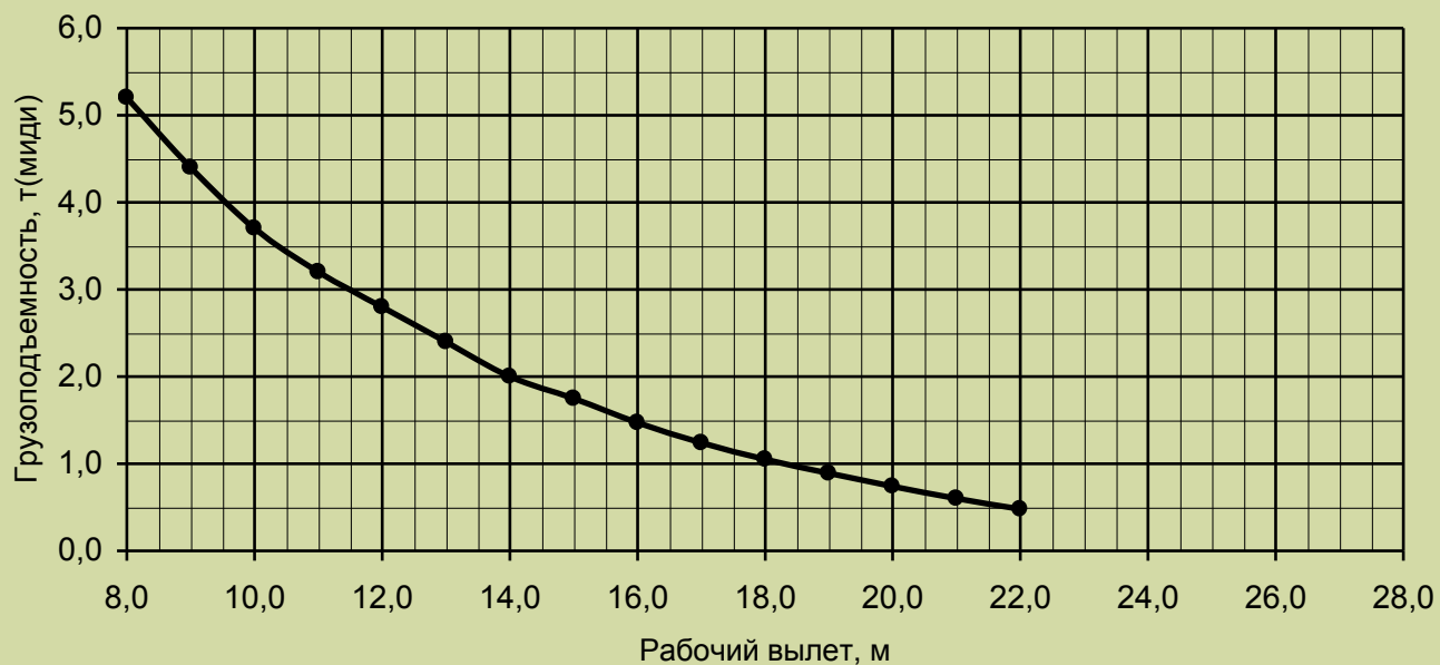
Грузовая характеристика Лст=9,9м. κ=10...12. Опорный контур 4,1х2,3м., противовес G=1,7т.
