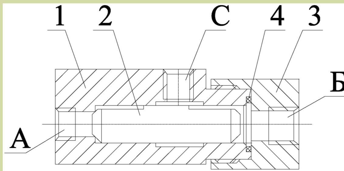
1- корпус; 2- золотник; 3- гайка; 4- уплотнение; А,В- напорные линии; С- к тормозу механизма поворота
