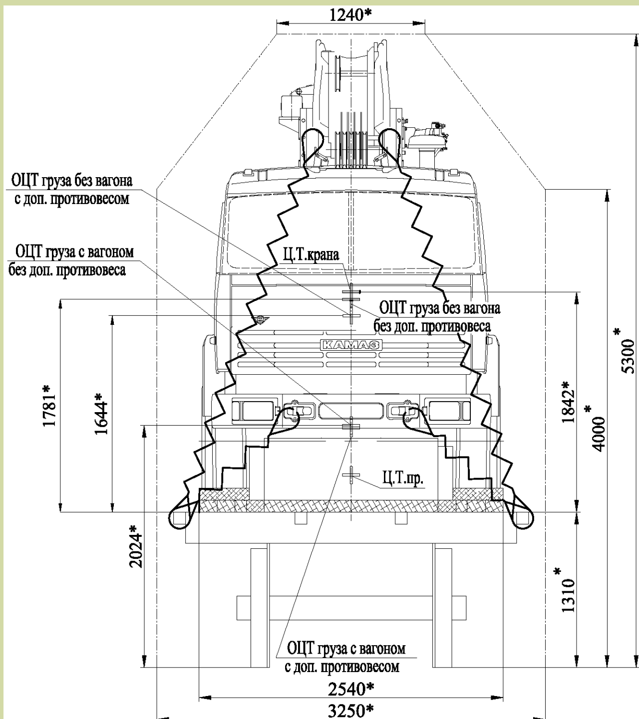
Рисунок 63 Перевозка крана железнодорожным транспортом
