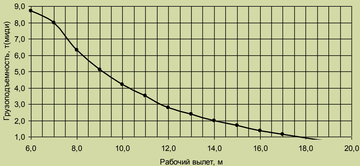
Грузовая характеристика. Лст=20,0-22,0м. \kappa=4 , противовес G=1,7 т.
