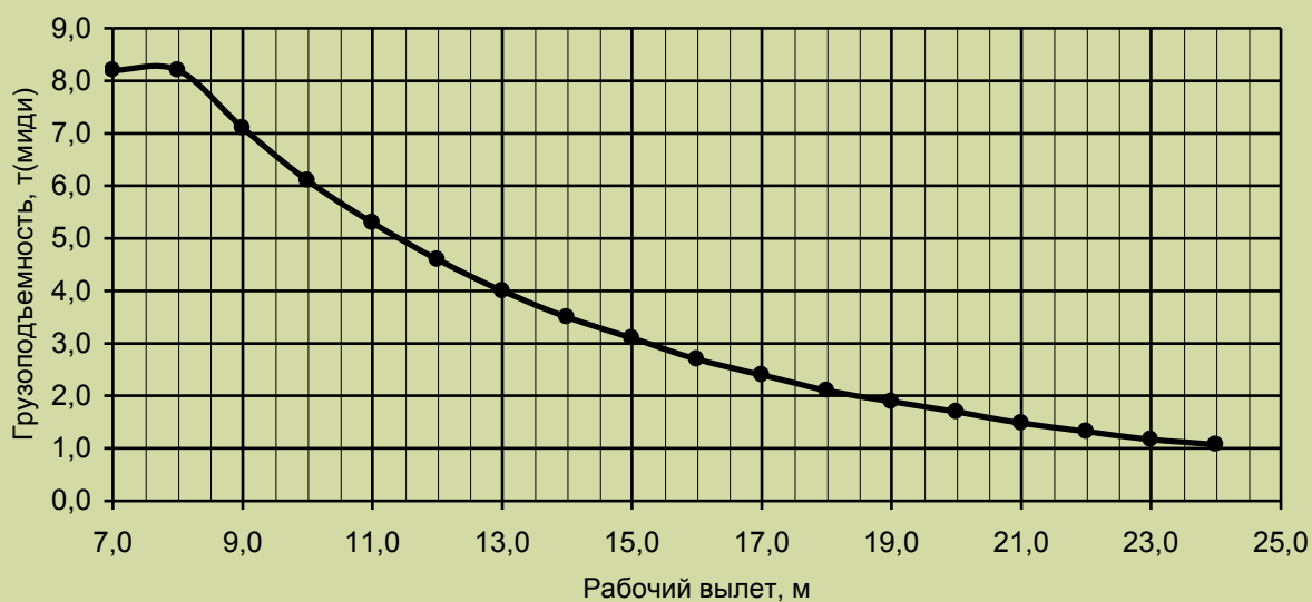
Грузовая характеристика. Лст=24,0-26,0м. \kappa=4 , противовес G=4,2 т.
