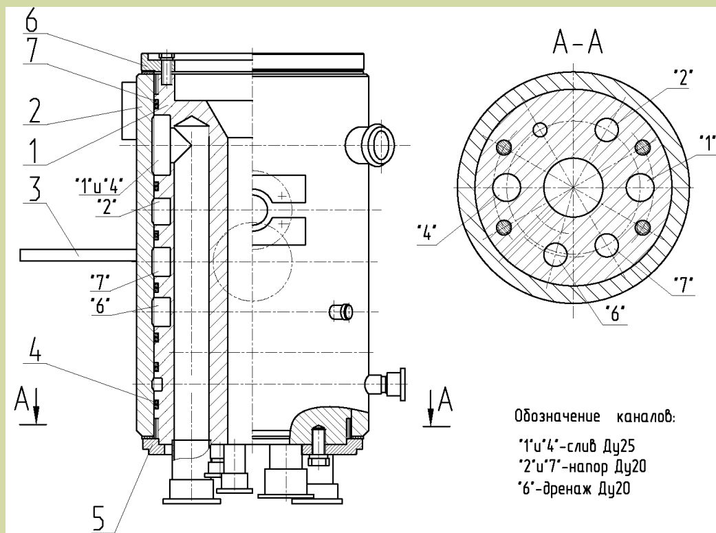
Рисунок 48 Центральный коллектор
