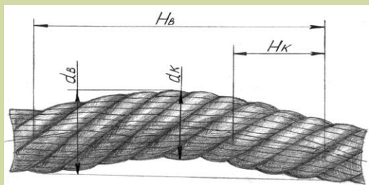
Волнистость каната
