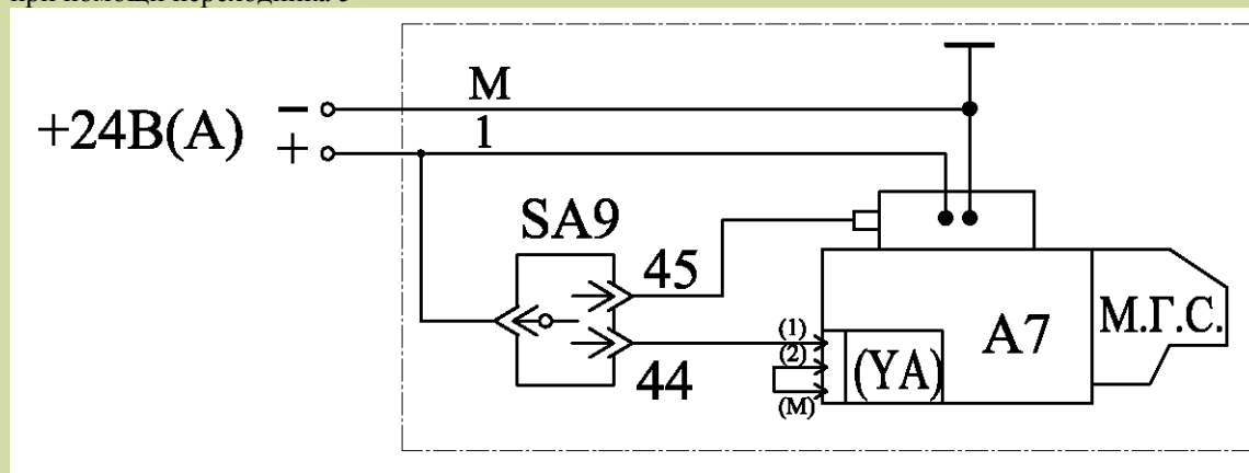
Рисунок 59 Электромонтажная схема подключения м.г.с.
