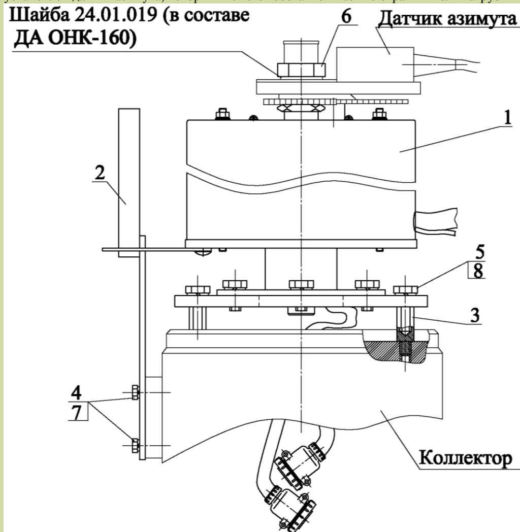
1 – токосъёмник; 2 – кронштейн; 3 – скоба; 4, 5 – болт; 6- гайка; 7,8 – шайба.
