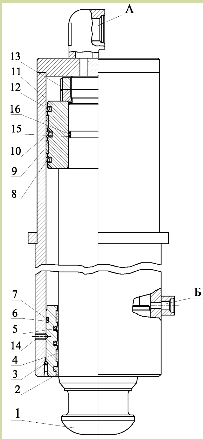
1 – шток; 2 – скребок; 3 – кольцо стопорное; 4 – кольцо направляющее; 5 – уплотнение стержневое; 6 – кольцо защитное; 7 – кольцо; 8 – уплотнение поршня; 9 – кольцо направляющее; 10 – уплотнение поршня; 11 – поршень; 12 – корпус; 13 – гайка; 14 – винт; 15 – кольцо защитное; 16 – кольцо А- отверстие поршневой полости; Б- отверстие штоковой полости
