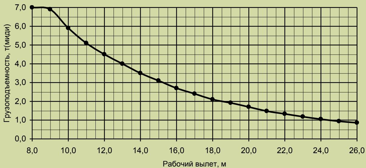
Грузовая характеристика. Лст=26,0-28,0м. \kappa=4 , противовес G=4,2 т.
