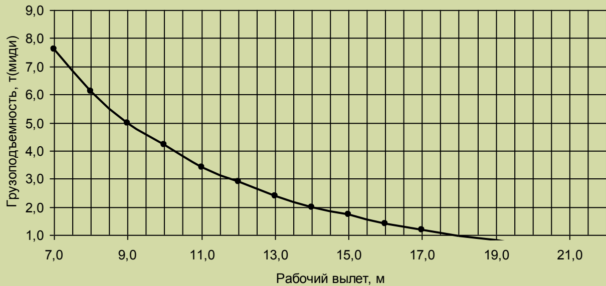
Грузовая характеристика. Лст=22,0-24,0м. \kappa=4 , противовес G=1,7 т.
