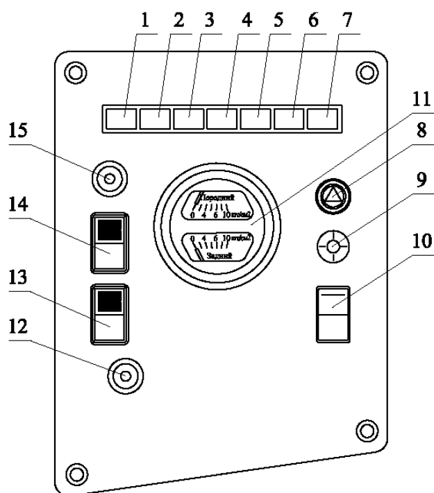
Рисунок 3 Дополнительная панель шасси МЗКТ-692340
