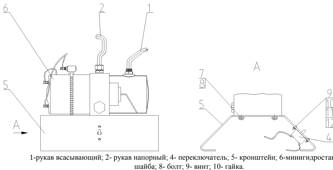
Рисунок 52 Минигидростанция в сборе
