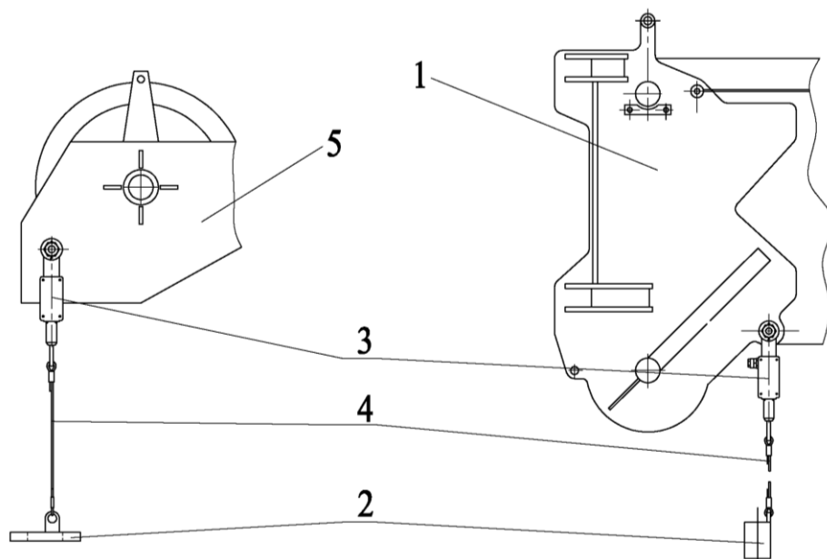
Рисунок 29 Ограничители высоты подъема
