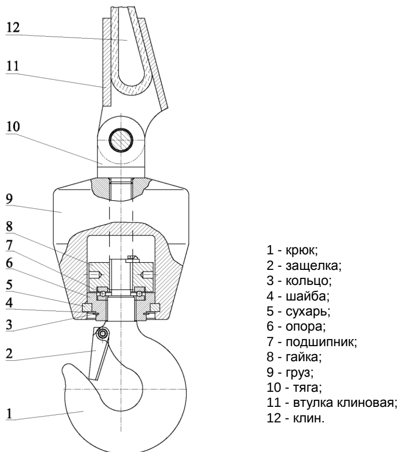
Рисунок 21 Обойма крюковая малая.
