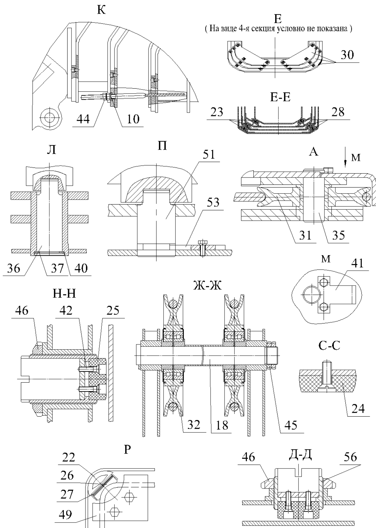
Рисунок 17.1 Стрела телескопическая
