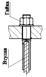
Схема заделки канатов механизма втягивания 4-й секции стрелы
