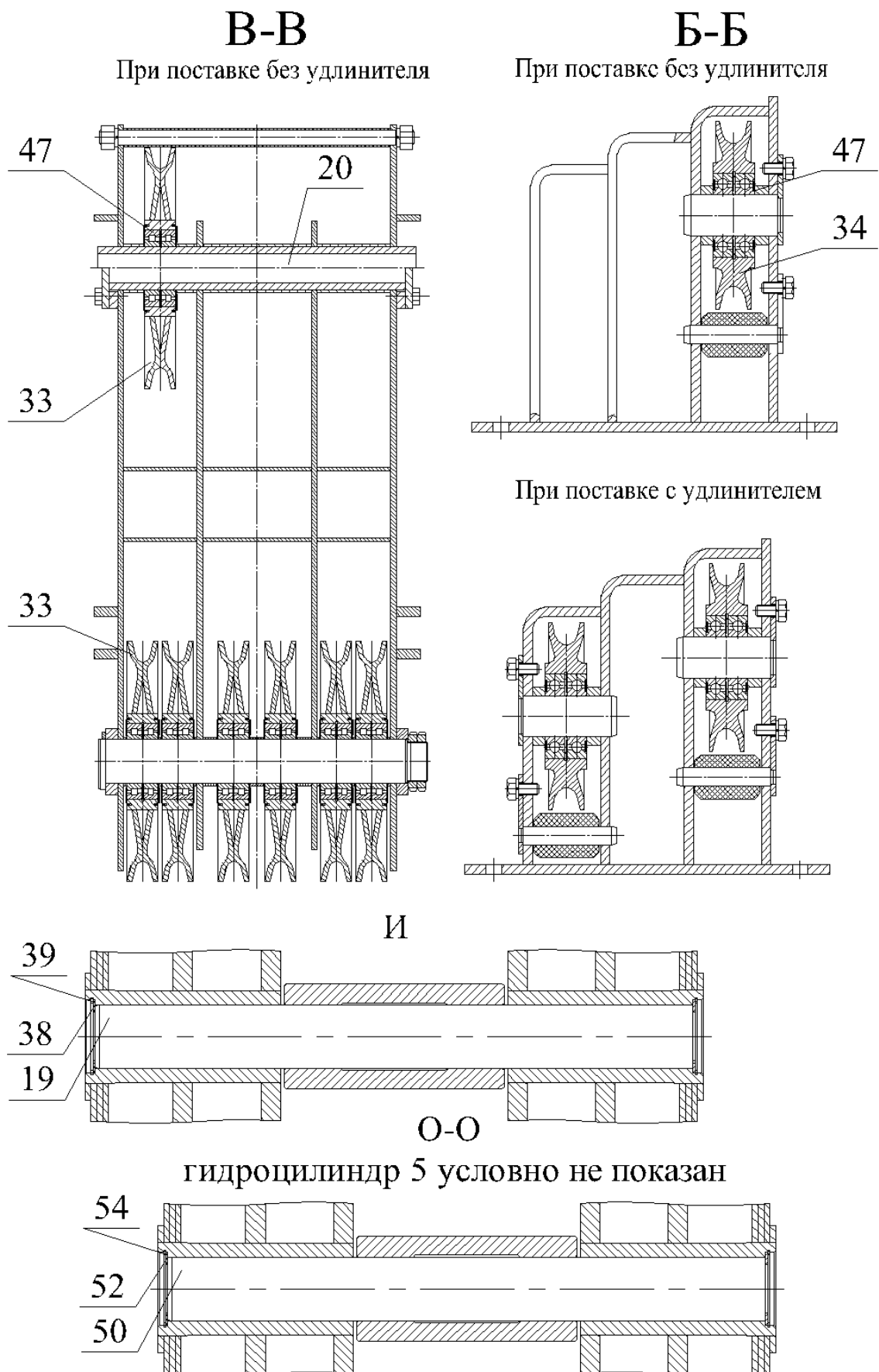
Рисунок 17.2 Стрела телескопическая
