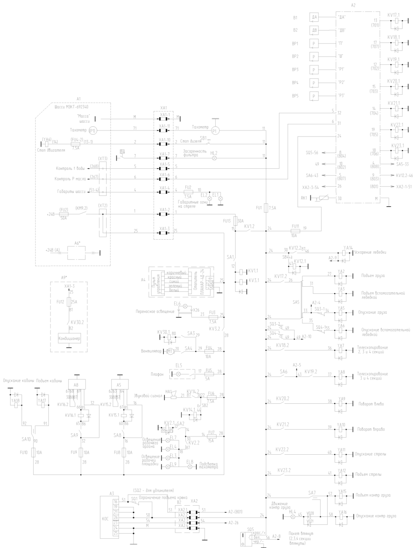
Рисунок 26 Схема электрическая принципиальная
