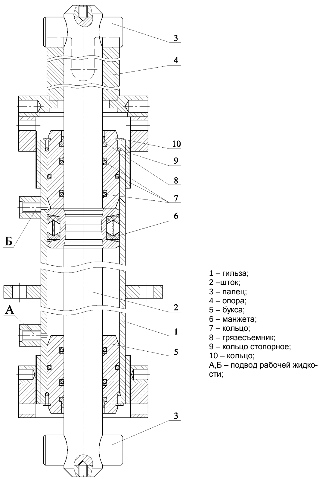
Рисунок 22 Гидроцилиндр установки дополнительных противовесов
