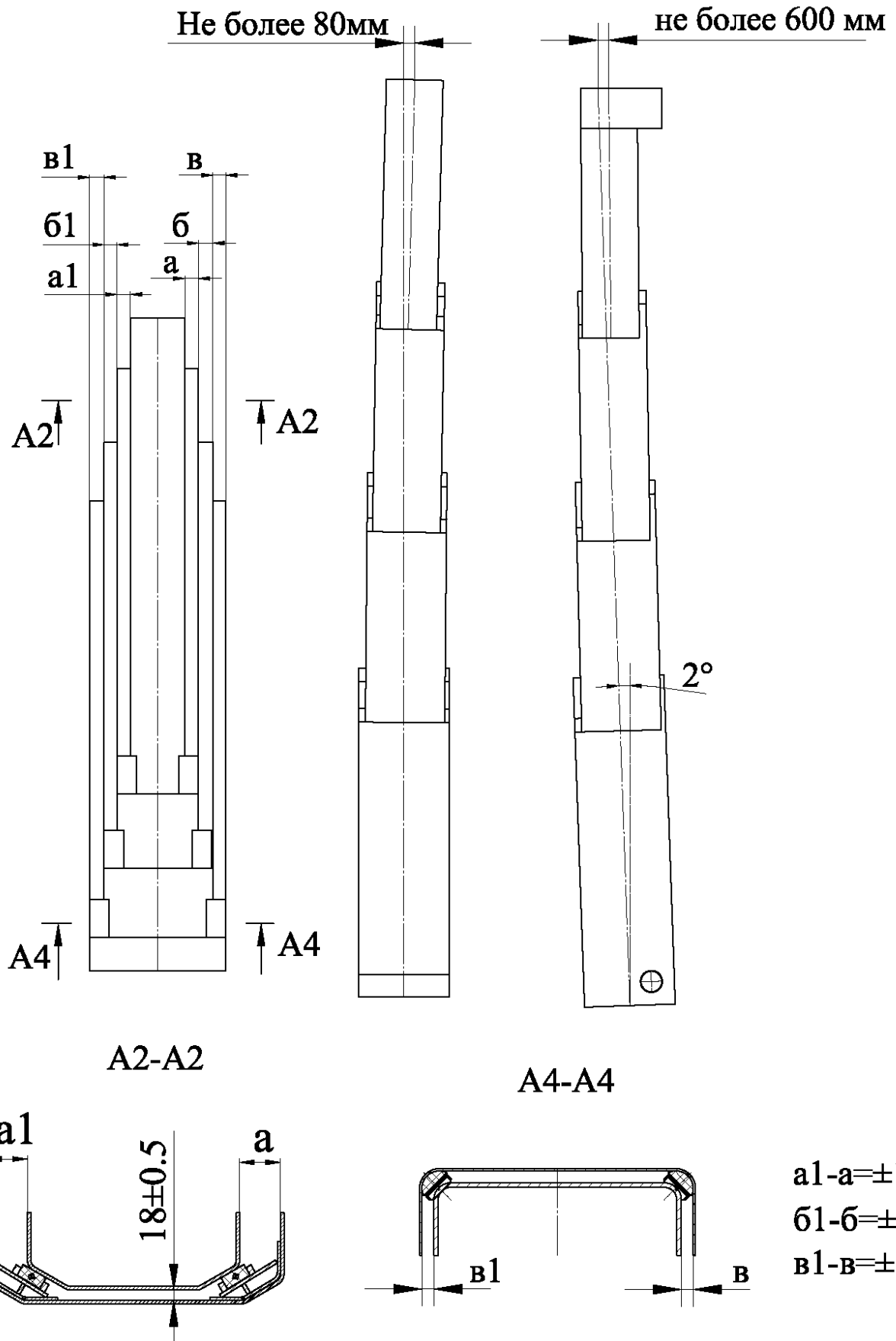
Рисунок 17.4 Схема регулировок отклонения секций от продольной оси.
