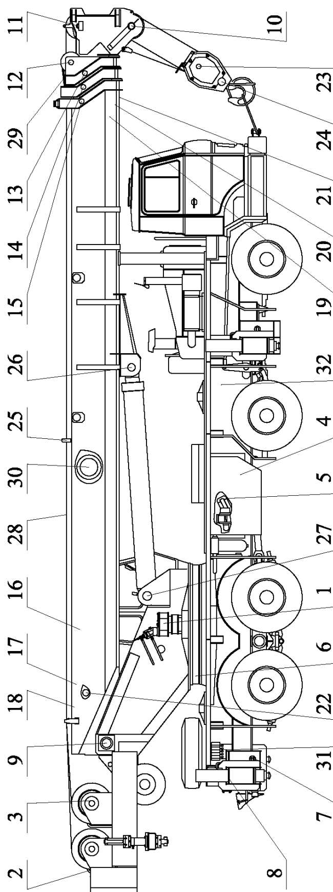
Рисунок 57 Схема смазки крана
