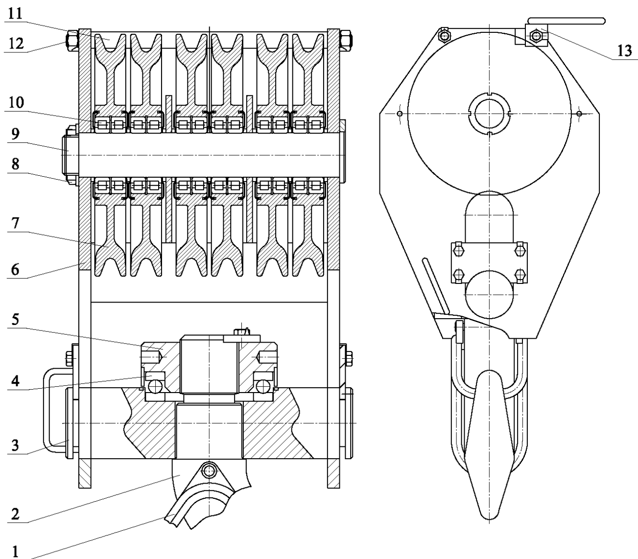
1 – скоба; 2 – крюк; 3 – траверса; 4,10 – подшипники; 5 – гайка; 6 – кожух; 7 – блок; 8 – гайка; 9 – ось; 11 – трубка распорная; 12 – шпилька; 13 – упор.
