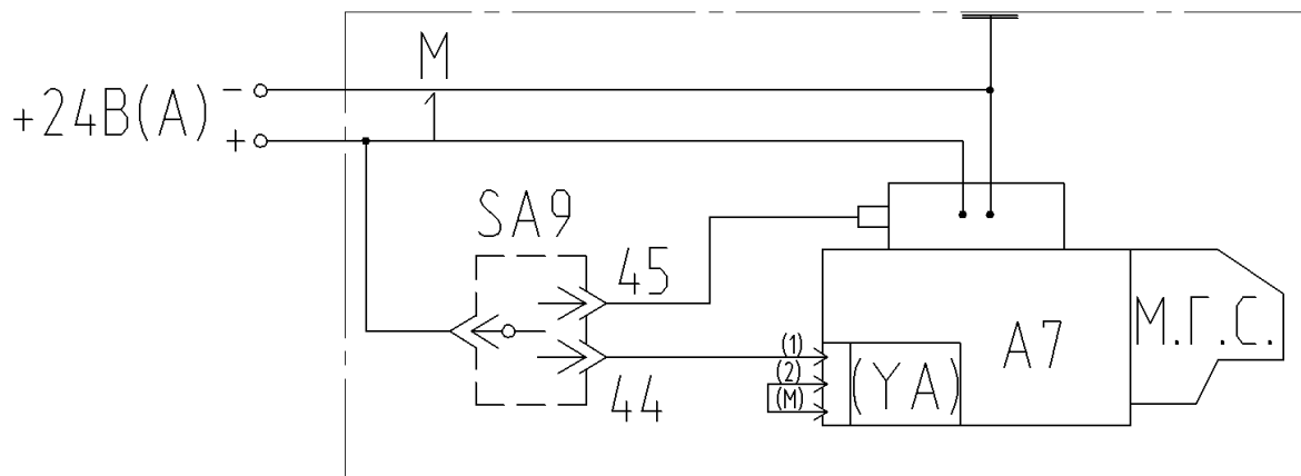
Рисунок 54 Электромонтажная схема подключения м.г.с.
