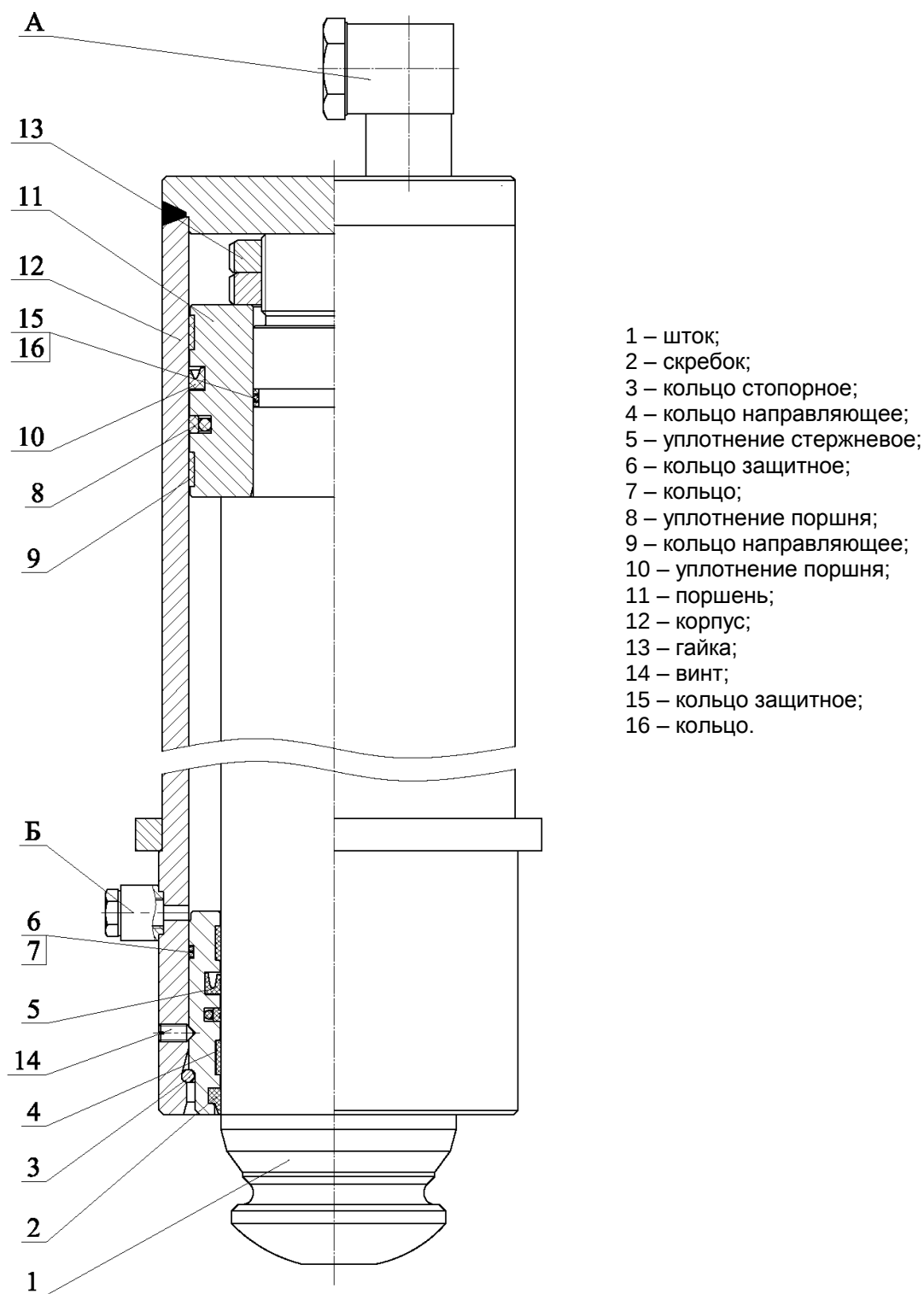
Рисунок 38 Гидроцилиндр опор
