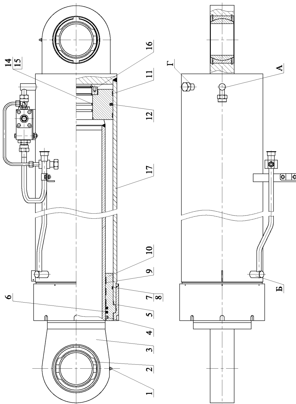
Рисунок 39 Гидроцилиндр подъема стрелы
