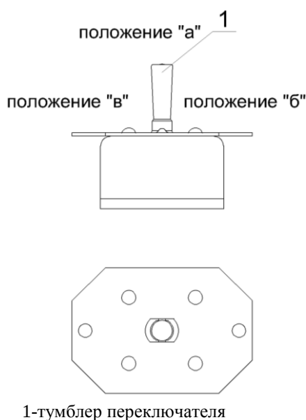
Рисунок 53 Переключатель
