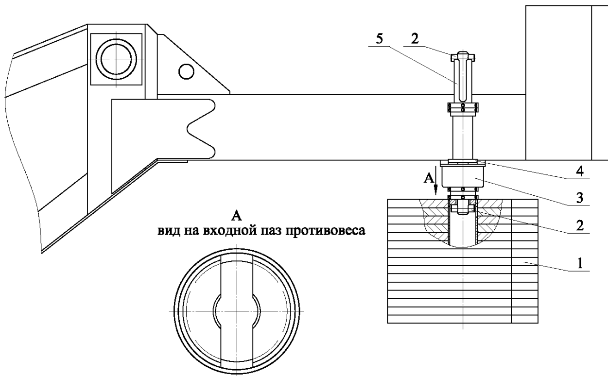
Рисунок 23 Установка дополнительного противовеса
