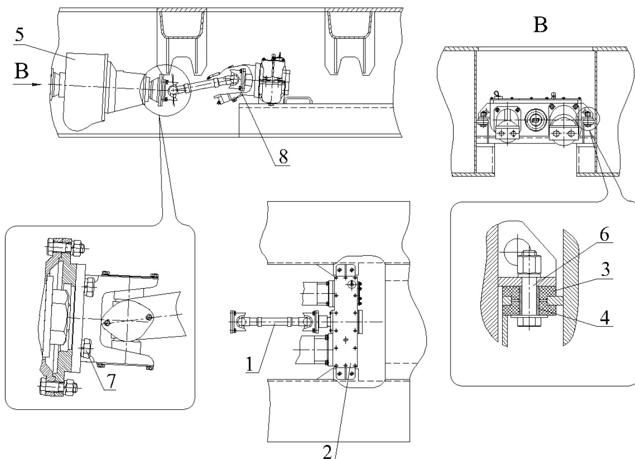
1 – карданный вал; 2 - редуктор с насосами; 3 – подушка; 4 – втулка; 5 – коробка отбора мощности; 6,7,8 – болты.
